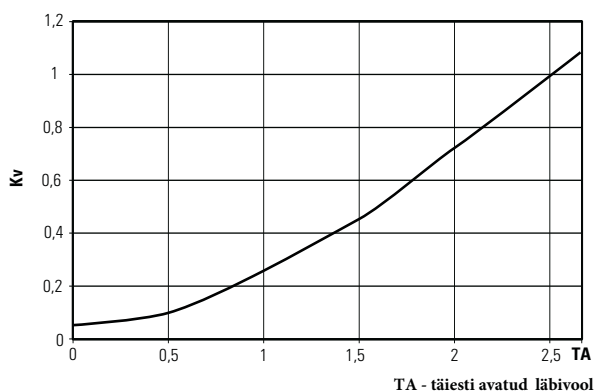
Rotameetri avatud asend (lahti pööratuna) ja KVS
