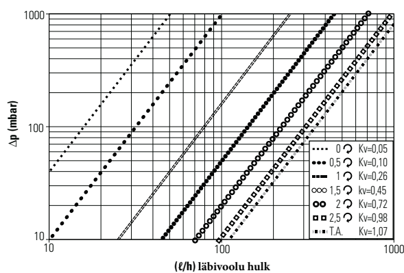
Rotameetri reguleerimine / KVS ja rõhu alanemine
